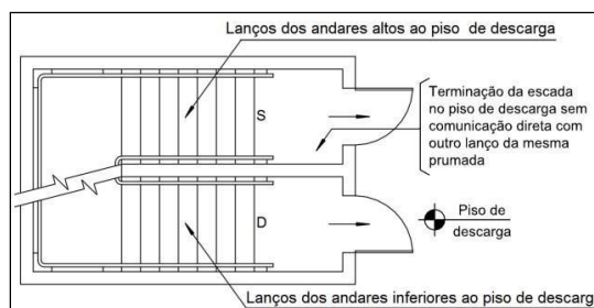
Figura 3 - Segmentação das escadas no piso da descarga
