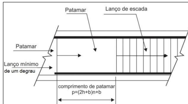
Figura 6 - Lanço mínimo e comprimento de patamar
