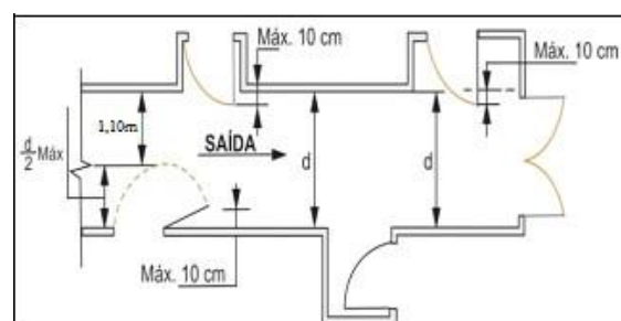
Figura2 - Abertura das portas no sentido de saída
